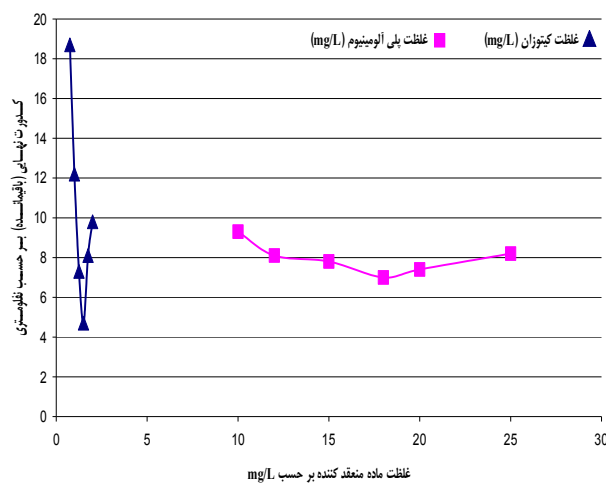
شکل شماره ۳. کارایی حذف کدورت در انواع و غلظت های مختلف منعقدکننده در کدورت اولیه ۵۰ واحد نفلومتری
